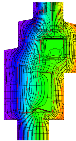
Isothermengrafik
